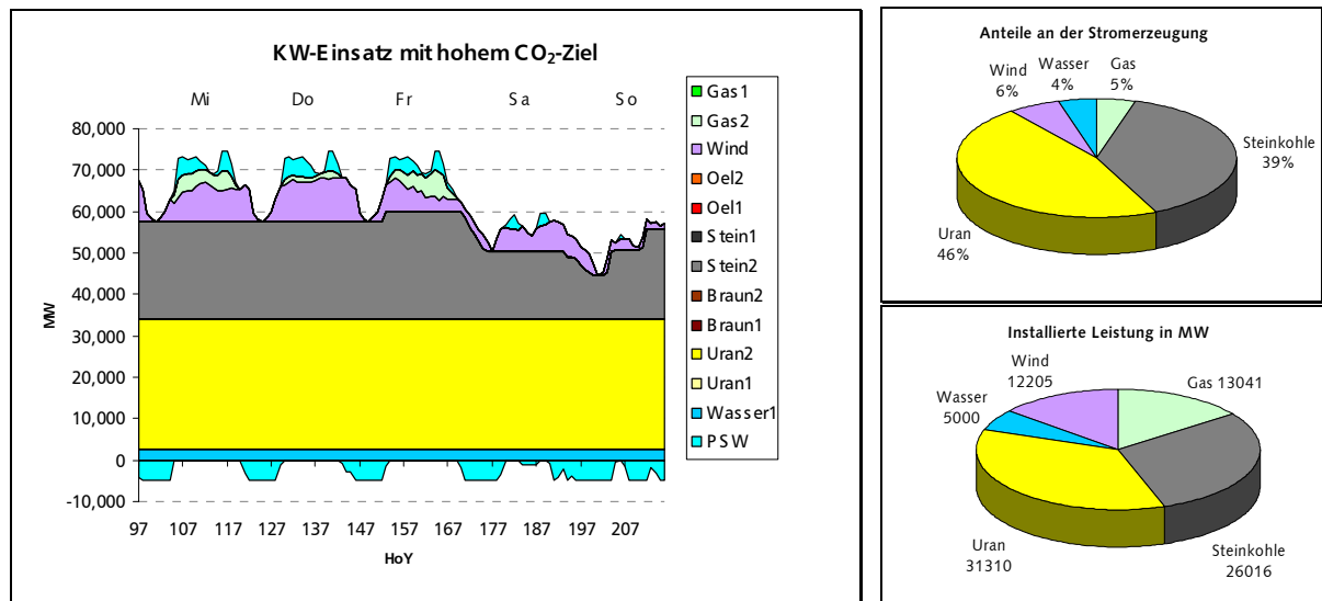
Bild 7.20: Verlauf des Kraftwerkseinsatzes und der Anteile der Stromerzeugung sowie der installierten Leistung 2020 mit völlig freier Zubaumöglichkeit und niedrigen Gaspreisen. Das Reduktionsziel ist hoch (-40%).
