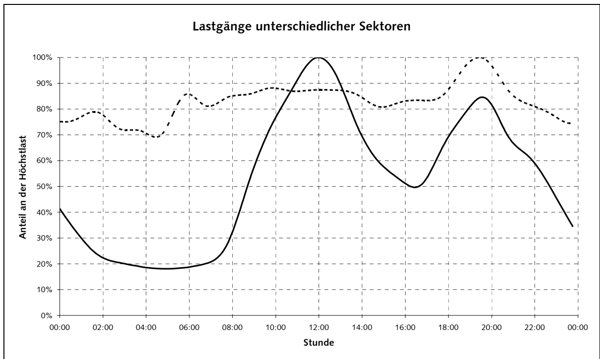
Bild 5.6: Vergleich des Nachfrageverlaufs von Haushaltskunden (durchgezogen) mit einem exemplarischen Verlauf der Last bei Gewerbe und Dienstleistern mit Kühlaggregaten, Büros, Schule u. ä. nach Vorgabe der Standardlastprofile (gestrichelt). Quelle: [VDEW02e].
