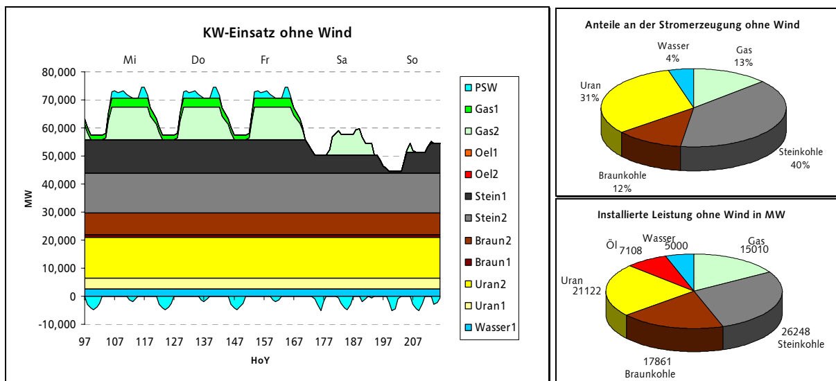
Bild 7.2: Von WEER berechneter Modellkraftwerkseinsatz für das Jahr 2000 ohne Windstromeinspeisung. Zur Deckung der Tagesspitzen werden die Pumpspeicherwasserkraftwerke (PSW) genutzt, die in der Nacht „geladen“ werden. Zu den Anteilen der nach PE-Trägern unterschiedenen Erzeugung siehe Text.
