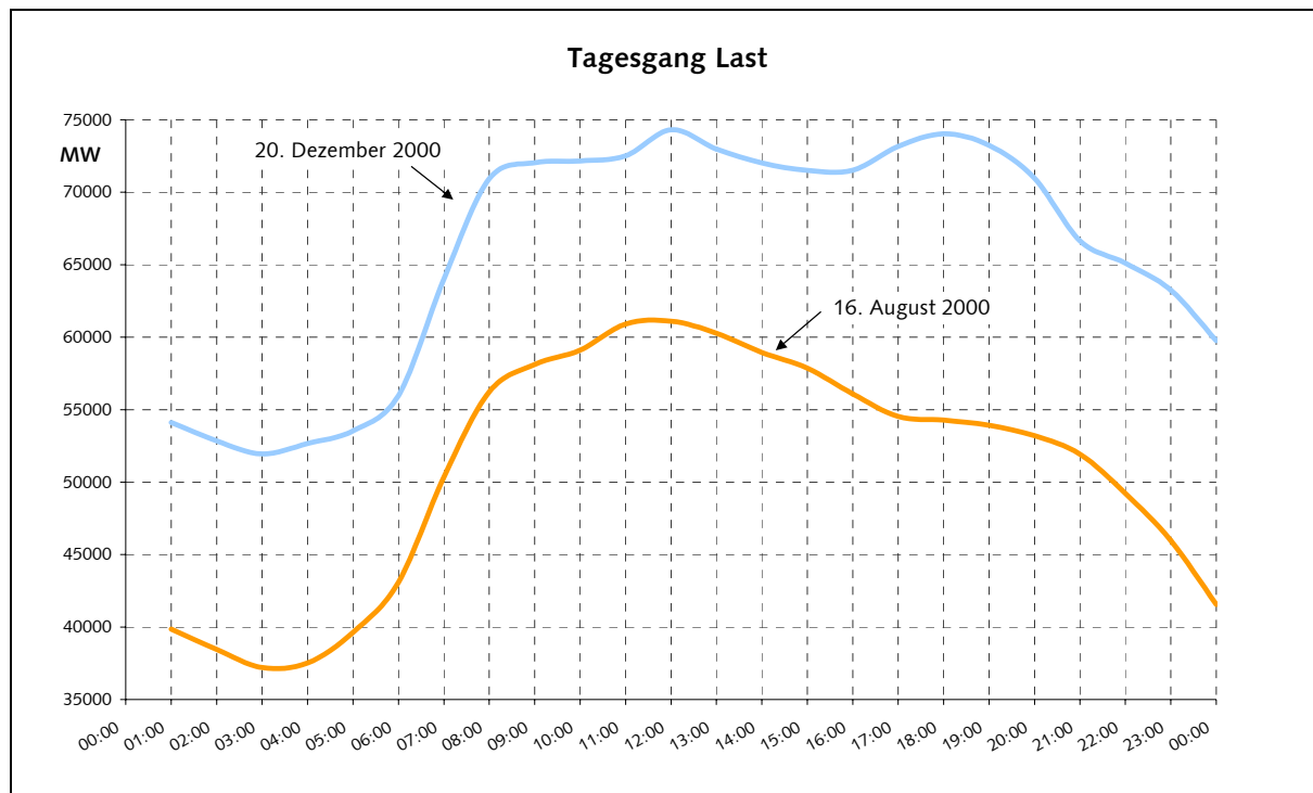
Bild 5.5: Verlauf der Nachfrage im deutschen Stromnetz an einem Sommer- und einem Wintertag 2000. Es handelt sich dabei um die zeitgleich addierten Verläufe der deutschen Übertragungsnetzbetreiber. Quelle: [UCTE01]
