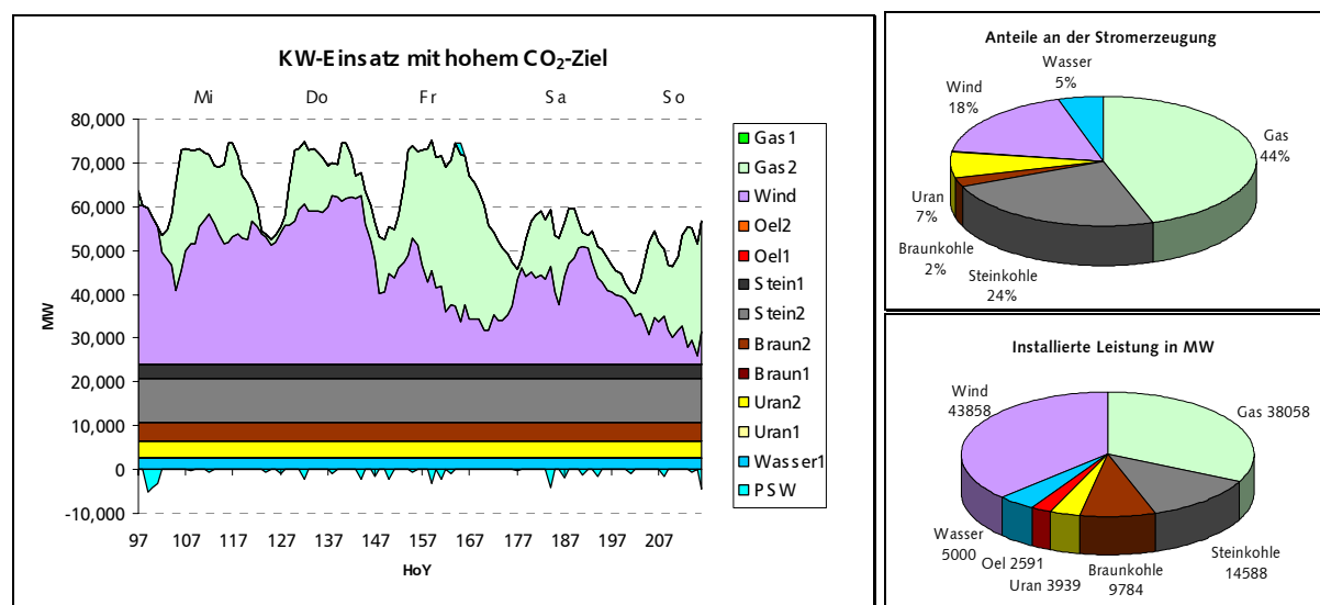
Bild 7.18: Verlauf der Stromerzeugung 2020 in einer exemplarischen Betrachtung einiger Tage sowie ganzjährige Anteile und installierte Leistung in einem Szenario, das WKA wie andere Erzeuger anhand der Kosten beurteilt. Gaspreis „hoch“, Klimaschutzziel hoch (-40%).
