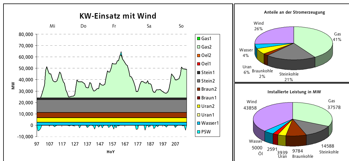
Bild 7.9: Durch WEsER-Optimierung berechneter konventioneller Kraftwerkseinsatz für 2020. Das Pumpspeicherwassersystem wird unregelmäßiger, besonders zur „Abfederung“ von Windstromerzeugungsspitzen genutzt.
