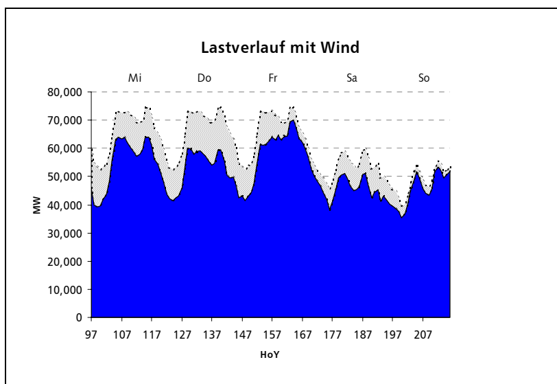
Bild 7.4: Verlauf der resultierenden Nachfrage (ausgefüllt) sowie der Einspeisung von Strom aus WKA (schraffiert) im Jahr 2010, aufgetragen über die Stunde des Jahres (HoY). Die obere, gestrichelte Begrenzungslinie gibt den unbeeinflussten Lastgang wieder.
