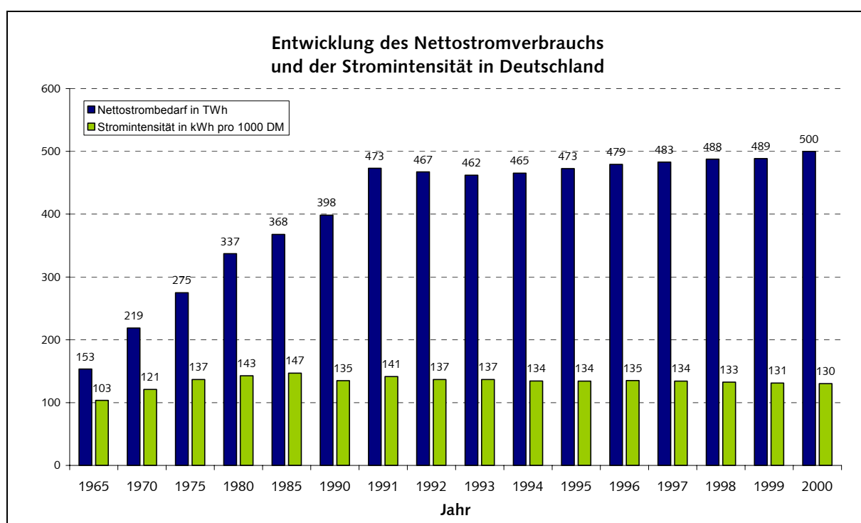
Bild 5.3: Nettostromverbrauch und Stromintensität im Vergleich. Bis einschließlich 1990 ohne DDR/neue Bundesländer. Quelle: [VIK02, BMWi01]
