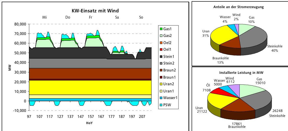
Bild 7.3: Von WEsER berechneter Modellkraftwerkseinsatz für das Jahr 2000 mit Windstromeinspeisung („realer“ Fall). Die Summe der Modellkraftwerksleistungen ergibt die resultierende Nachfrage (Nachfrage – Windeinspeisung).
