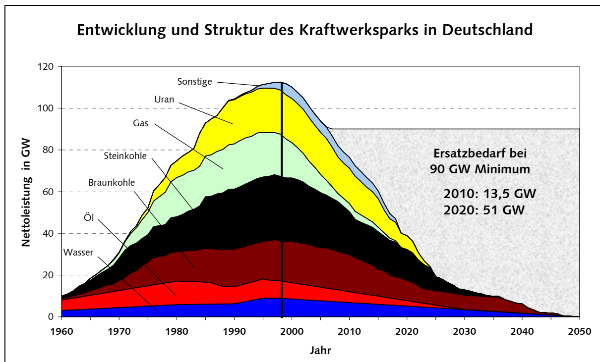
Bild 4.7: Entwicklung der installierten konventionellen Kraftwerksleistung in Deutschland bis 2050. Quellen: [BEI00, Markewitz99, Heithoff00]
