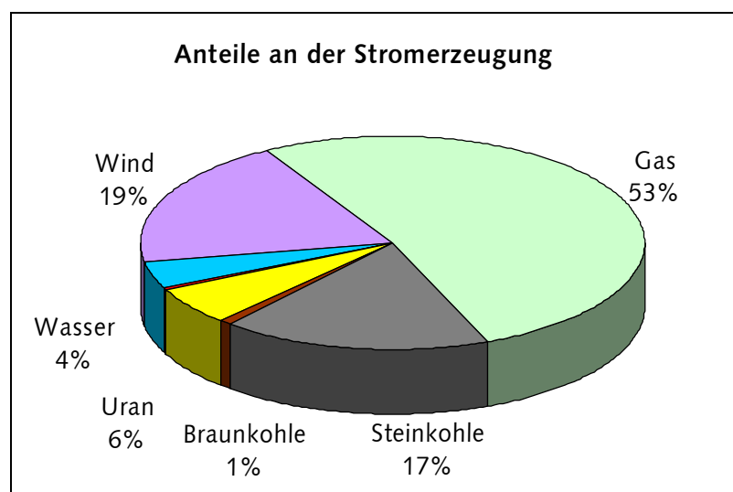
Bild 7.12: Zusammensetzung der für das Jahr 2020 erforderlichen Stromerzeugung bei der Annahme einer aufgrund eines schlechten Windjahres verringerten Windstromerzeugung bei Einhaltung des 40% CO 2 -Reduktionsziels.
