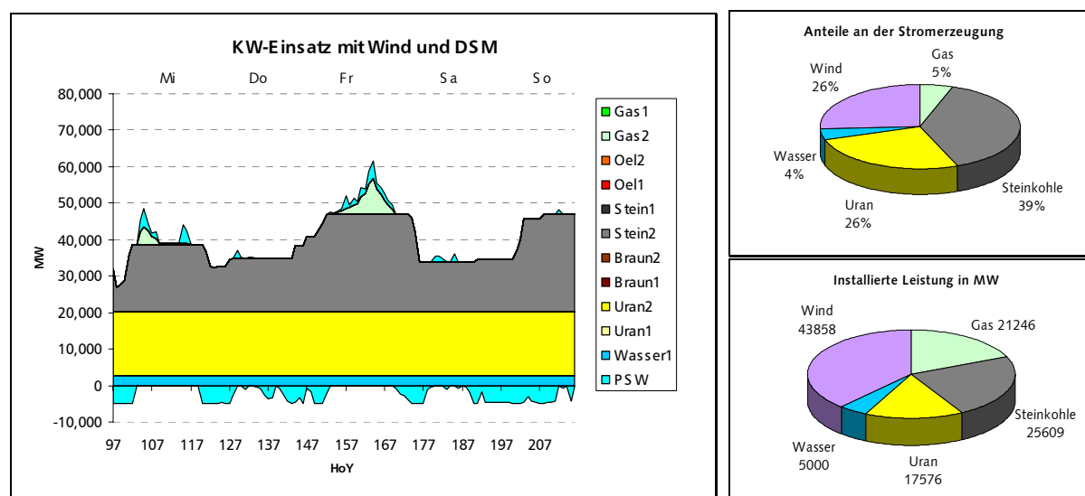
Bild 7.16: Einfluss des demand side management bei der Optimierung ohne Vorgabe oder Beschränkung von installierter Leistung. Der Gasanteil in der Erzeugung wird nochmals deutlich reduziert.
