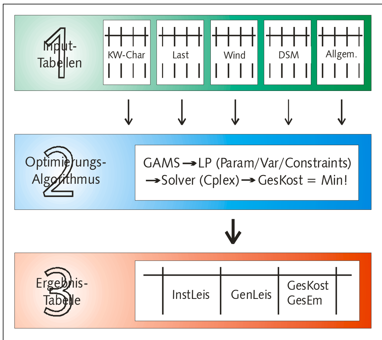
Bild 6.1: Struktur des Modells WesER. Im Teilbereich 1 werden die Daten in Form von Tabellen zur Verfügung gestellt. Im zweiten Abschnitt erfolgt die Optimierung im GAMS/CPLEX-System, im Teilbereich 3 werden die Ergebnisse ausgegeben und aufbereitet.
