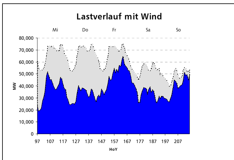
Bild 7.8: Verlauf der resultierenden Nachfrage (ausgefüllt) sowie der Einspeisung von Strom aus WKA (schraffiert) im Jahr 2020, aufgetragen über die Stunde des Jahres (HoY). Die obere, gestrichelte Begrenzungslinie gibt den unbeeinflussten Lastgang wieder.
