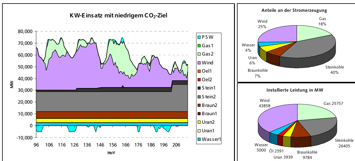
Bild 7.19: Ergebnis der WEER-Optimierung mit der im Vergleich zu Bild 7.18 veränderten Voraussetzung eines niedrigeren CO 2 -Reduktionsziels (-21%).
