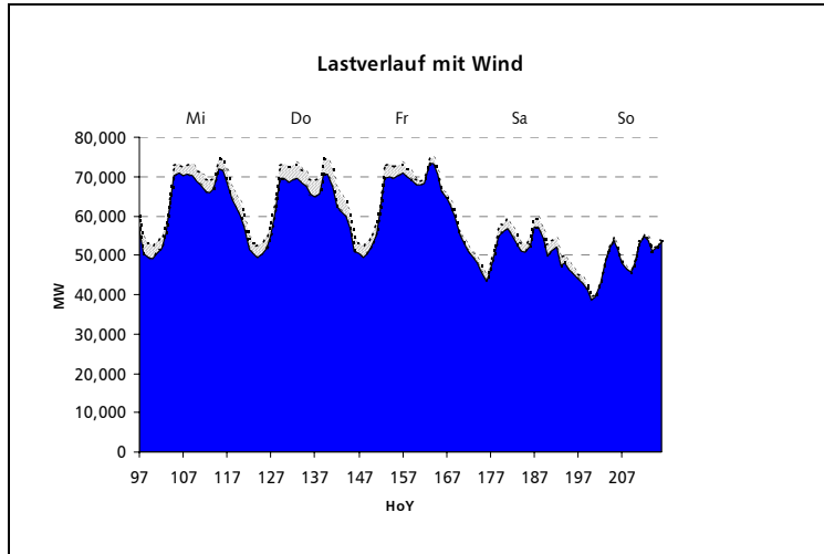
Bild 7.1: Verlauf der resultierenden Nachfrage (ausgefüllt) sowie der Einspeisung von Strom aus WKA (schraffiert) im Jahr 2000, aufgetragen über die Stunde des Jahres (HoY). Die obere, gestrichelte Begrenzungslinie gibt den unbeeinflussten Lastgang wieder.
