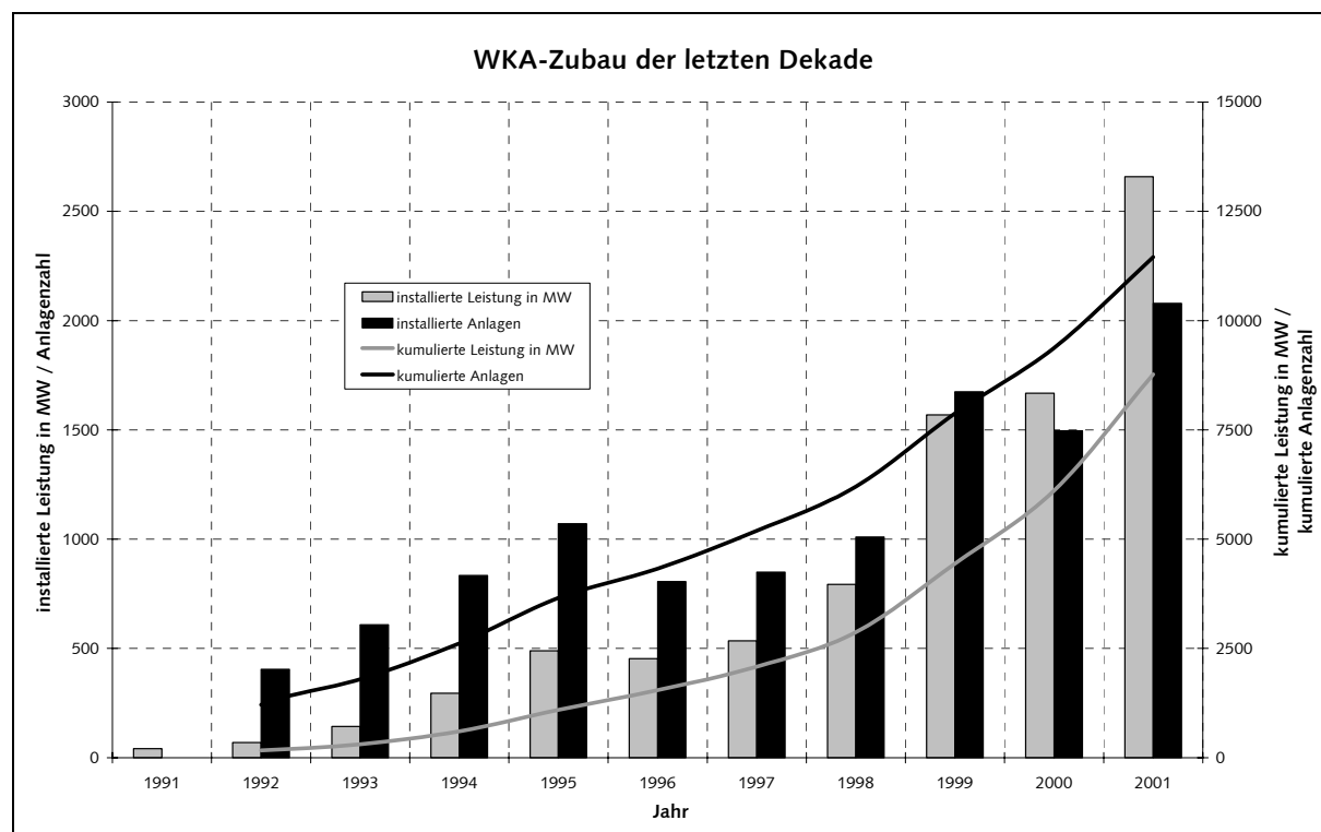
Bild 3.1: Jährliches und kumuliertes Wachstum der WKA-Zahl und der installierten Leistung der letzten 10 Jahre. Quelle: [BWE02].
