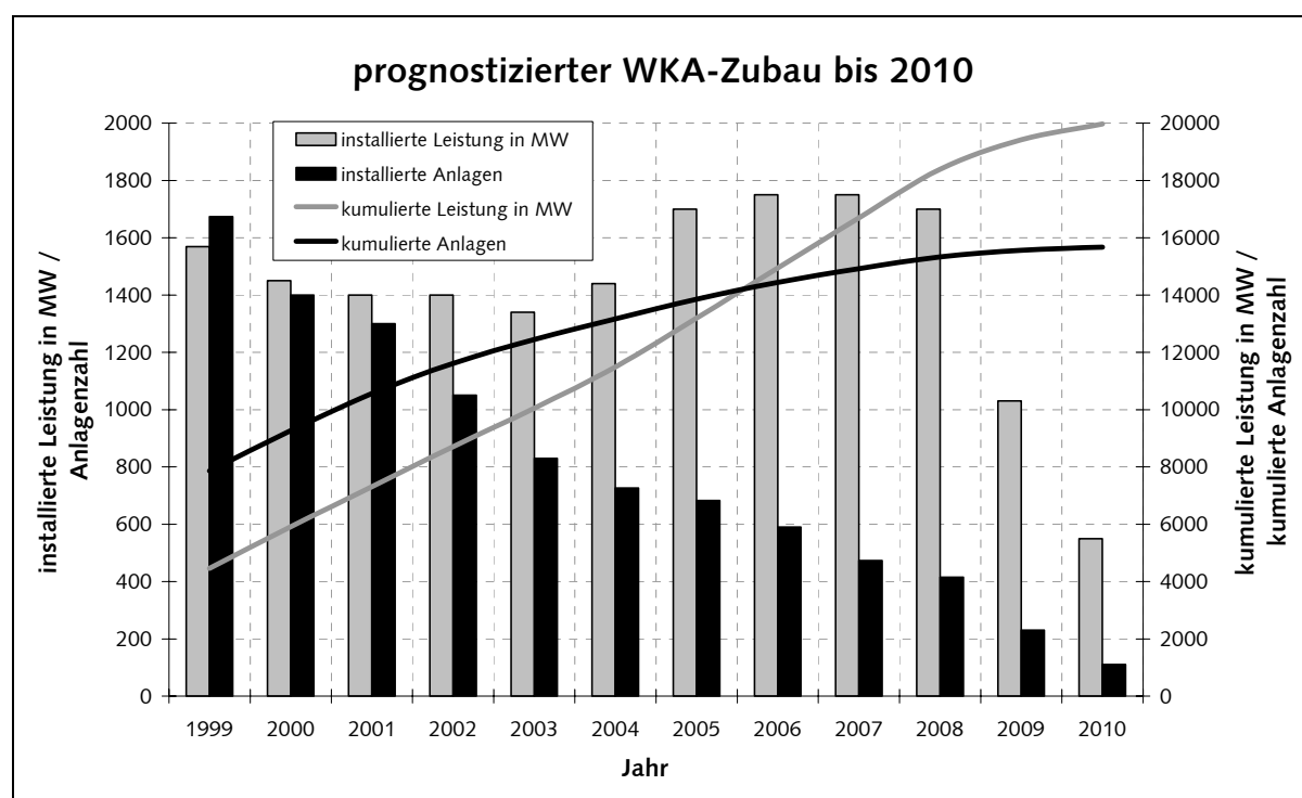
Bild 3.4: Entwicklung der WKA-Leistung und –Anlagenzahl bis 2010 nach einer Analyse des BMWi. Die Prognose aus dem Jahr 1999 wurde bereits durch die Zubau-Zahlen 2000 und 2001 von der Realität überholt. Quelle: [Mayer00].
