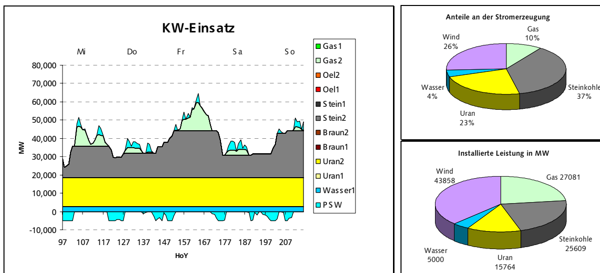
Bild 7.15: WEER-Ergebnis für die Bestimmung eines kostenoptimierten konventionellen Kraftwerksparks und -einsatzes für 2020 unter der Annahme eines hohen Gaspreises, normaler Windstromerzeugung, der Erreichung des CO 2 -Reduktionsziels sowie keiner Einschränkung oder Vorgabe einer installierten konventionellen Leistung.
