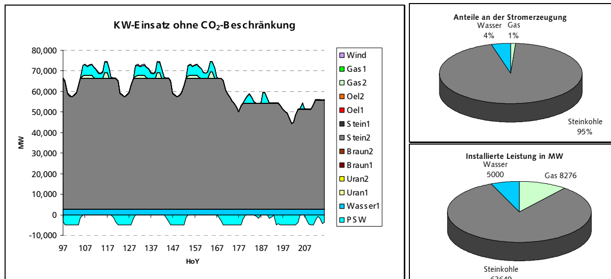
Bild 7.21: Optimierungsergebnis ohne die Vorgabe eines CO 2 -Reduktionsziels.
