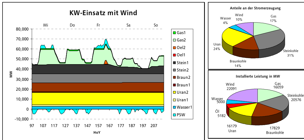
Bild 7.5: Durch WEsER berechneter Kraftwerkseinsatz sowie Anteile an der Stromerzeugung und installierte Leistung für das Jahr 2010. Aufgrund einer Vollbenutzungsstundenzahl von weniger als 2300 bei den WKA, ist der Anteil an der installierten Leistung (21%) deutlich höher als bei der Erzeugung (10%).
