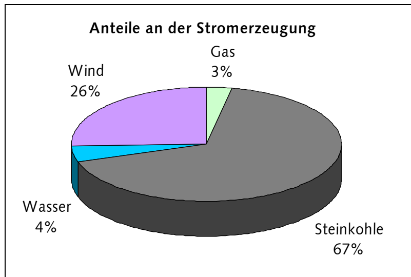
Bild 7.17: Anteile an der Stromerzeugung im Falle einer uneingeschränkten Einsatz- und Zubaumöglichkeit der Modellkraftwerke bei Verzicht auf Erreichung des Klimaschutzziels, jedoch unter Einbeziehung des Windstroms. Der Gaspreis ist „hoch“.
