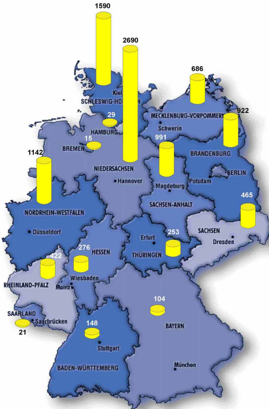
Bild 3.3: Installierte Leistung an WKA in den Bundesländern, Stand Juni 2002. Angaben in MW. Quelle: [REISIO2].
