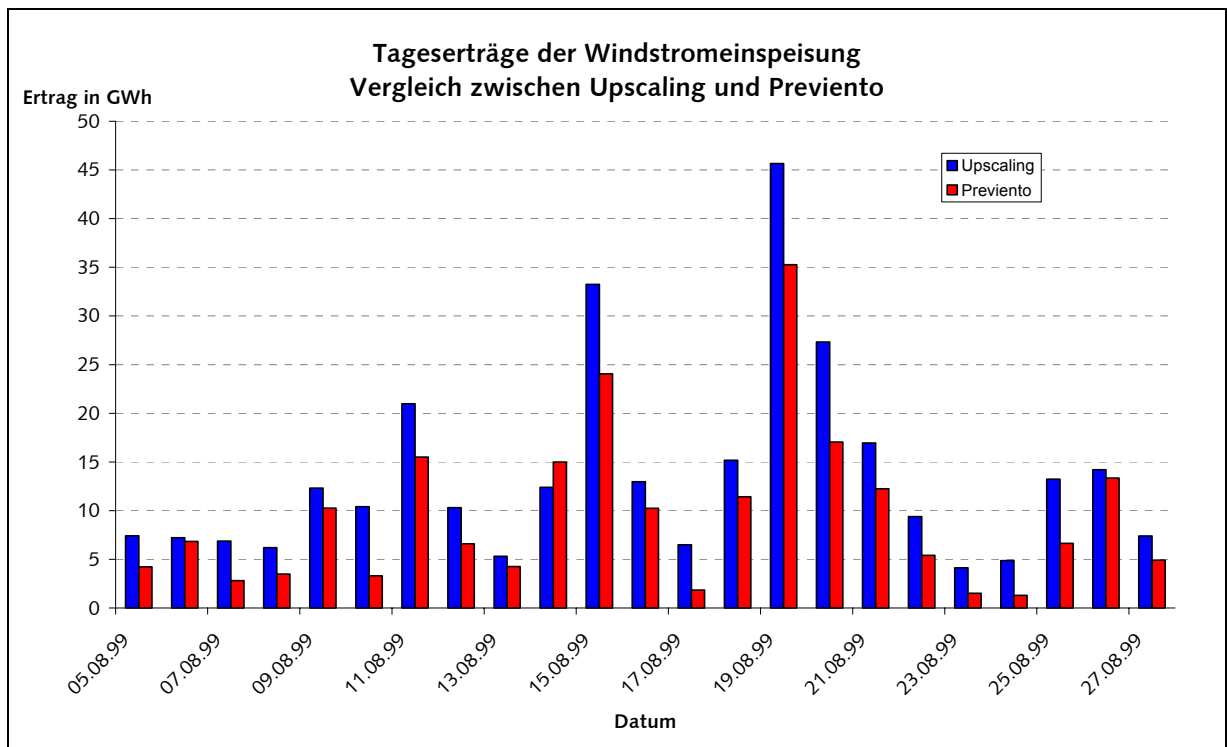
Bild 3.9: Vergleich der erzielten Tagessummen durch Upscaling-Methode und Previento-Vorhersage. Die Ursache der geringeren Werte der Previento-Vorhersage sind im Wesentlichen in der schon erwähnten nächtlichen Unterschätzung der Stromspeisung zu finden.
