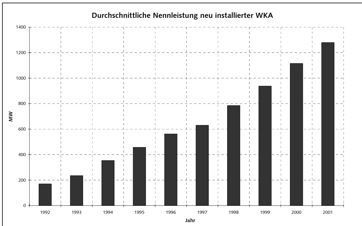
Bild 3.2: Steigerung der durchschnittlichen Anlagengröße neu installierter WKA während der letzten 10 Jahre. Quelle: [BWE02].
