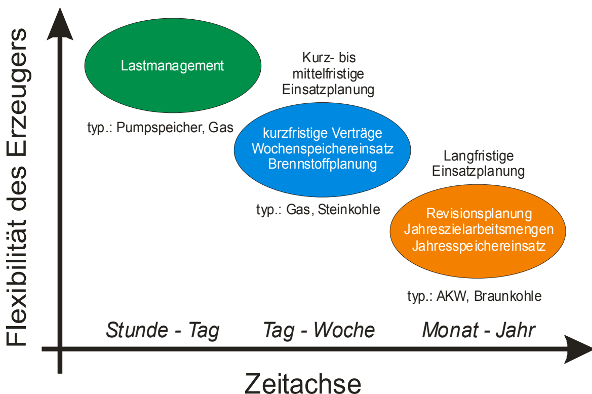
Bild 4.5: Schematische Darstellung der Kraftwerkseinsatzplanung von Stromerzeugern unterschiedlicher Flexibilität. Üblicherweise wird „von rechts nach links“ geplant, die „Grundlast“ also zuerst abgedeckt.
