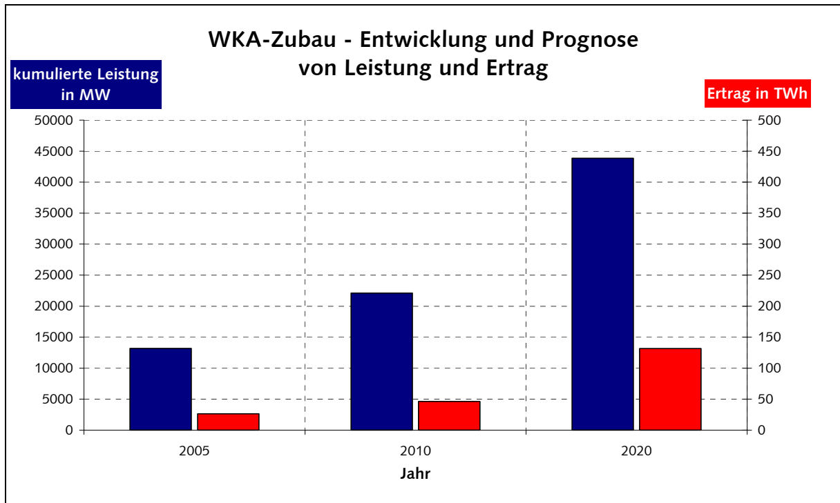
Bild 3.5: Prognostizierte Entwicklung der kumulierten Leistung an WKA in Deutschland bis 2020. Der Ertrag ist für ein durchschnittliches Windjahr angegeben und könnte 2020 25% des Strombedarfs decken. Quelle: [DEWI02].
