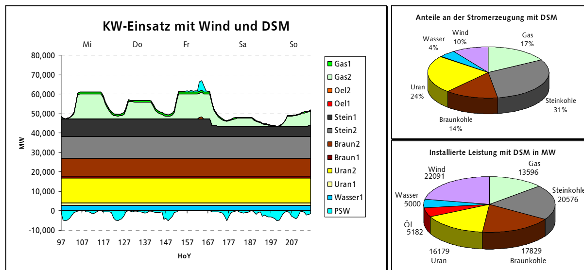
Bild 7.6: Anwendung von DSM zur Vergleichmäßigung der resultierenden Nachfrageganglinie. Während sich die Anteile an der Erzeugung nicht ändern, verringert sich die zugebaute Leistung an Gaskraftwerken nahezu um den Maximalbetrag des DSM.
