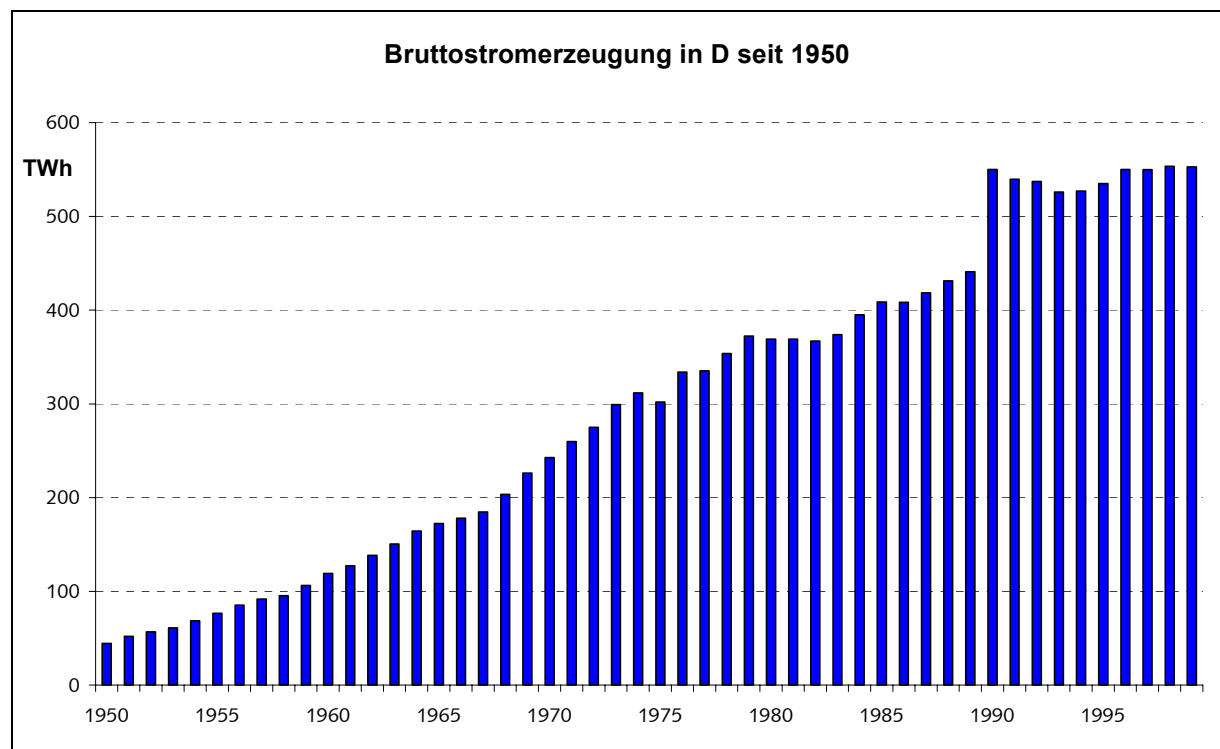
Bild 4.1: Entwicklung der Stromerzeugung in D seit 1950. Ab 1990 inkl. neue Bundesländer. Quelle: [DEBRIV02, BMWi01].
